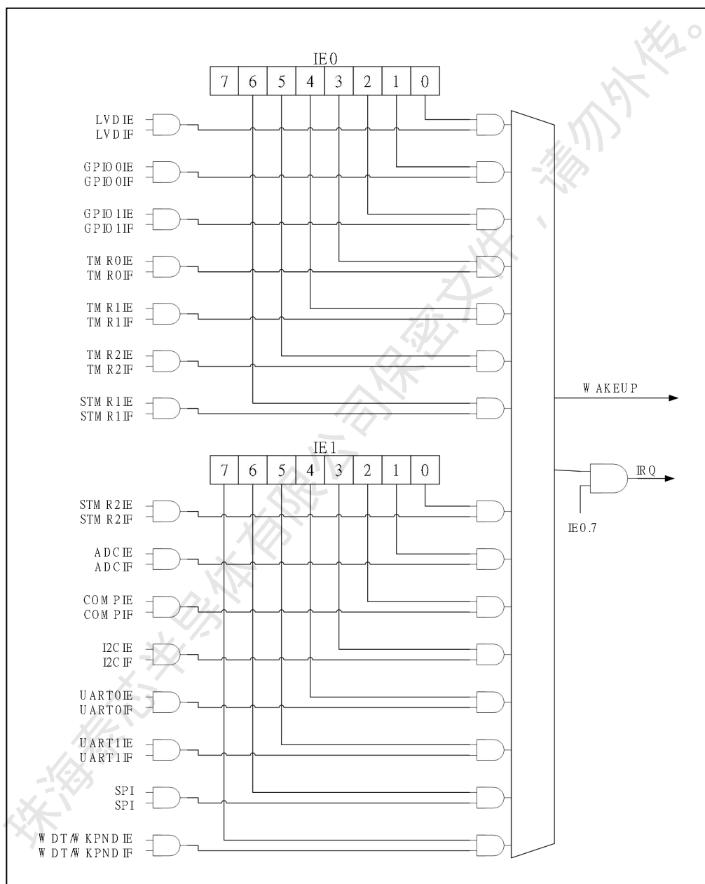
图 8-1 中断结构图
