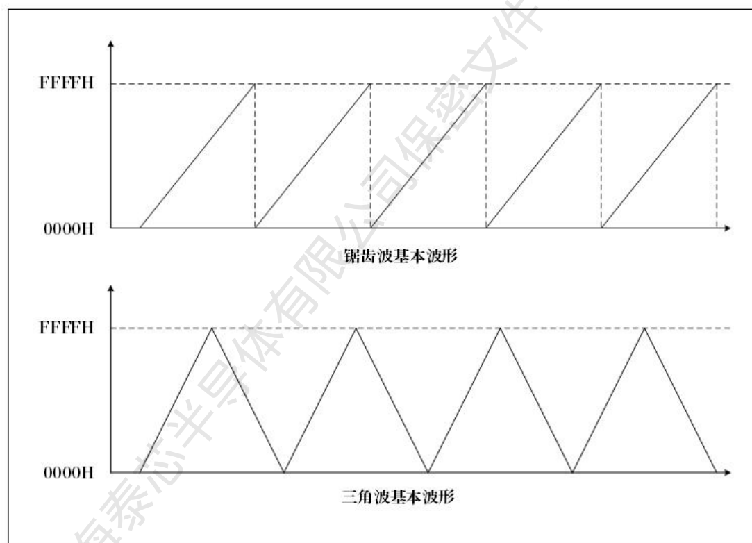
图 15-1 基础波形图
